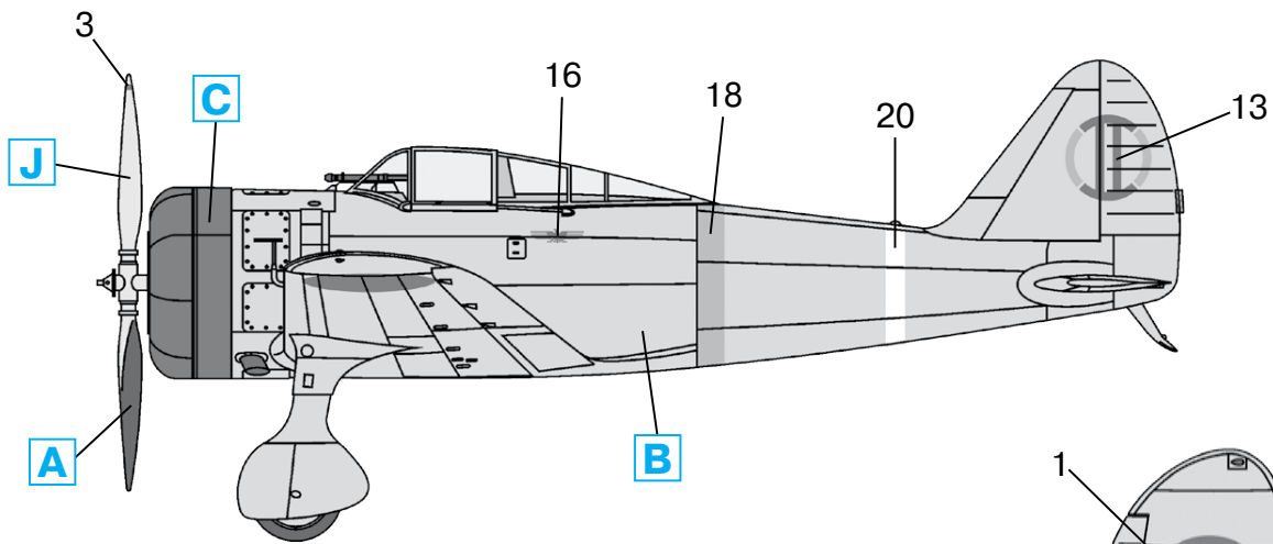
Ки-27б, сержант Сигэру Такува, 64-й полк, 1-я эскадрилья, Халхин-Гол, август 1939 г. Ki-27b, Sergeant Shigeru Takuwa, 64. Sentai, 1. Chutai, Nomonhan, August 1939
