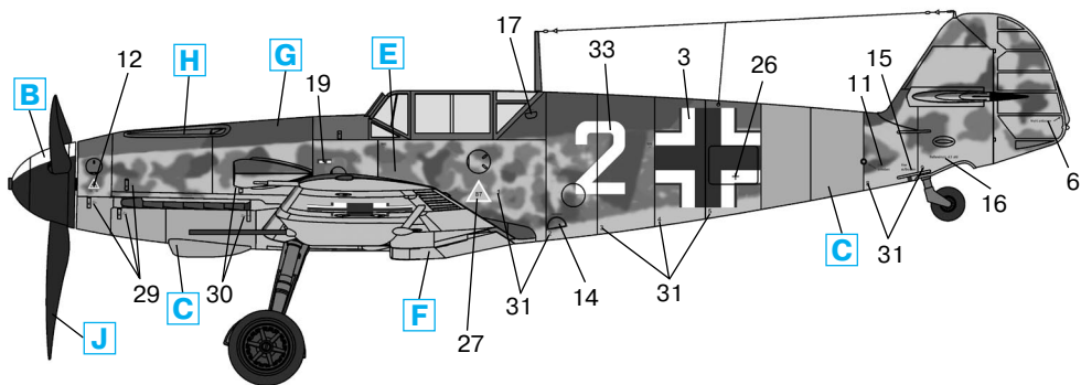
Мессerschмитт Bf 109F-4/R6, I./JG 52, район Кубани, июнь 1942 г. Messerschmitt Bf 109F-4/R6, I./JG 52, Cuban area, June 1942
