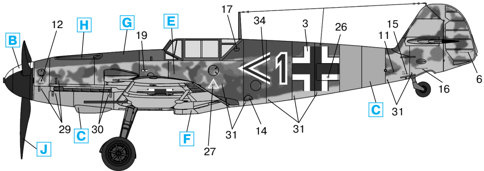
Мессerschmitt Bf 109F-4/R6, I./JG 52, район Кубани, июнь 1942 г. Messerschmitt Bf 109F-4/R6, I./JG 52, Cuban area, June 1942
