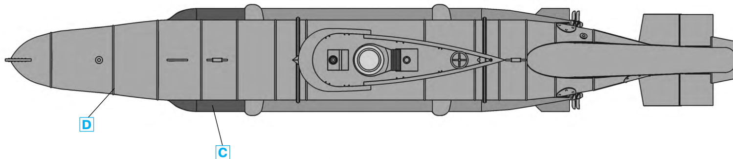
U-Boat Type XXVIIB Seehund, Lehrkdo 300, Surendorf, May 1945. Подводная лодка типа XXVIIB "Seehund", учебная команда 300, Зурендорф, май 1945 г.
