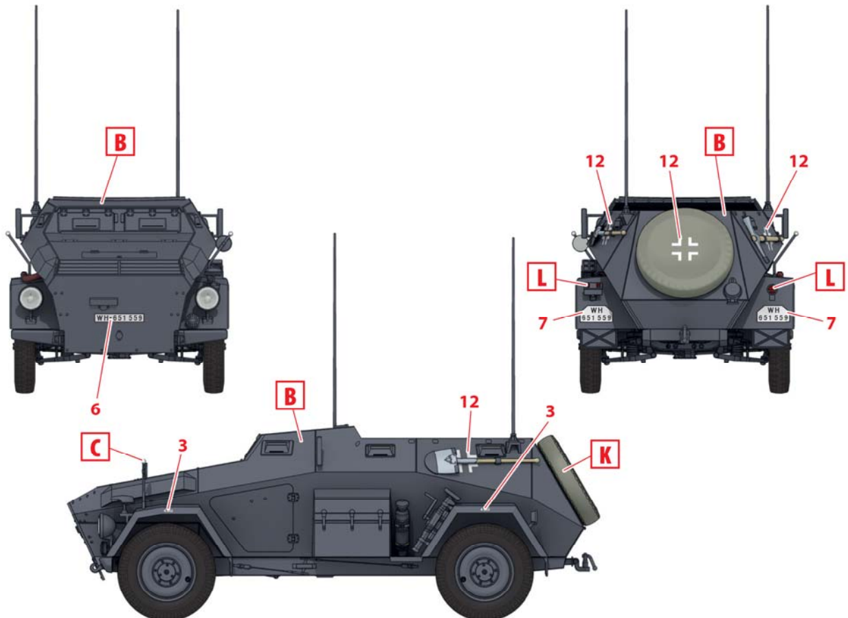
2. Sd.Kfz. 247 Ausf.B, Россия, осень 1941 г. Sd.Kfz. 247 Ausf.B, Russia, Autumn 1941
