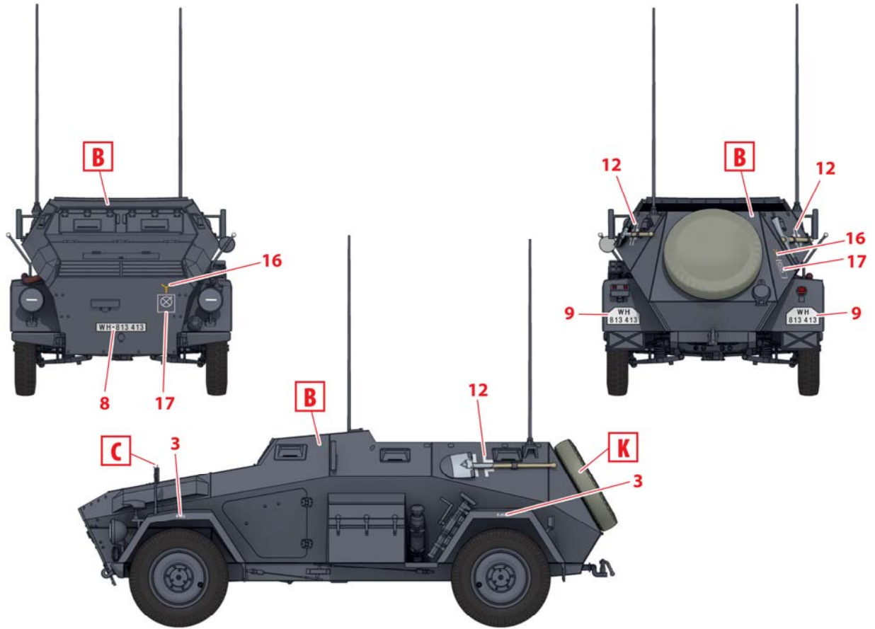
3. Sd.Kfz. 247 Ausf.B, 7-я танковая дивизия, Россия, лето 1941 г. Sd.Kfz. 247 Ausf.B, 7th Pz.D., Russia, Summer 1941
