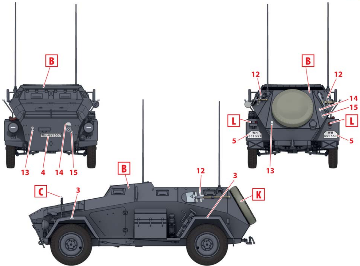
1. Sd.Kfz. 247 Ausf.B, дивизия Grossdeutschland, Украина, лето 1942 г. Sd.Kfz. 247 Ausf.B, Grossdeutschland division, Ukraine, Summer 1942
