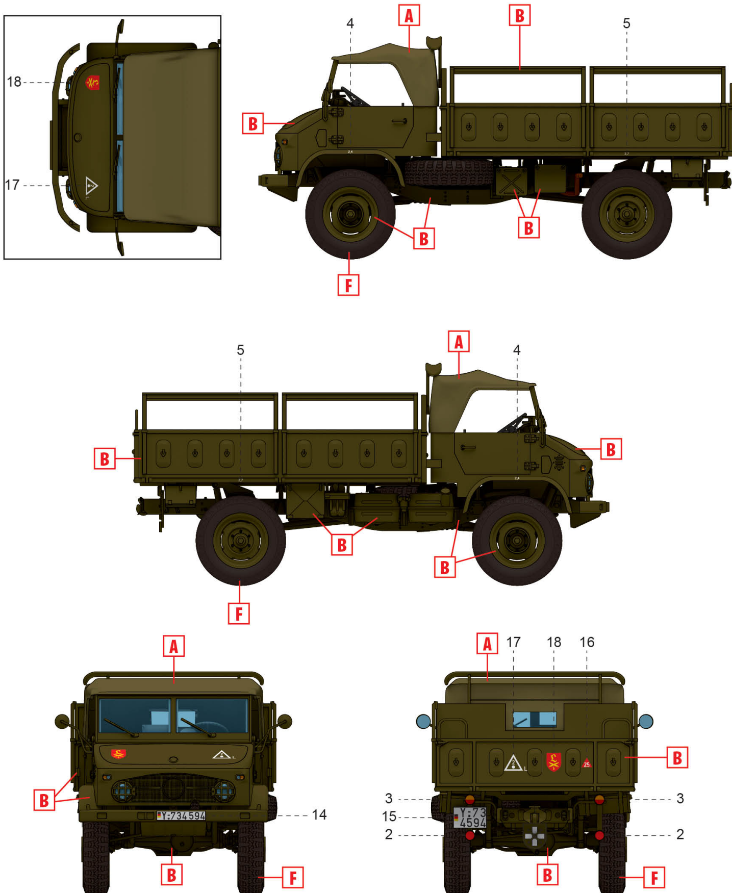
3. Unimog S 404, 5-й учбовий артилерійський полк, Ідар-Обрештайн, 1970-ті роки Unimog S 404, 5th Artillery Training Regiment, Idar-Obrestein, 1970s
