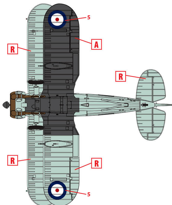
4. Gloster Sea Gladiator Mk.II, Хал Фар, Мальта, червень 1940 р. Gloster Sea Gladiator Mk.II, Hal Far, Malta, June 1940
